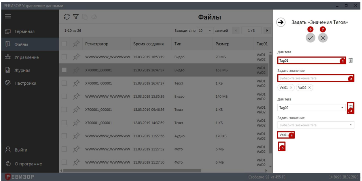
Рисунок 39 – Задание «Значений Тегов» для «Файла»/«Файлов»
