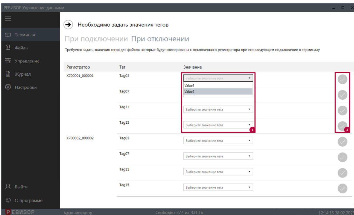
Рисунок 24 – Задание «Значений Тегов» при подключении регистратора
