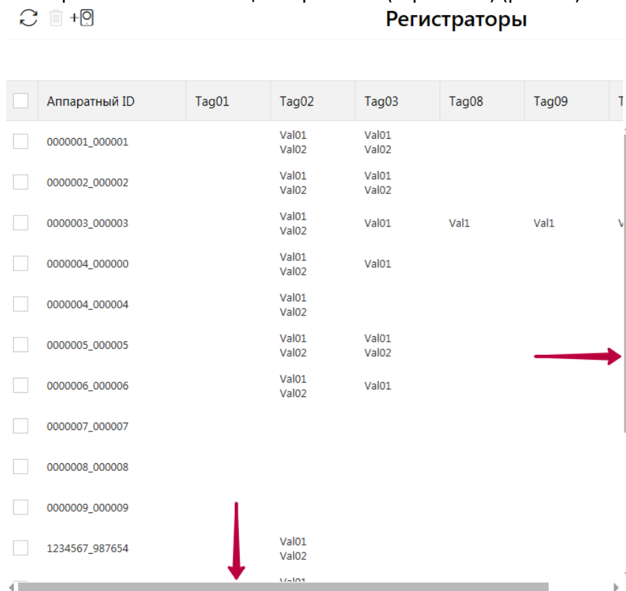
Рисунок 79 – Позиционирование списка «Регистраторов»
